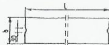
Rys. 1. Wymiarowanie krawężników
