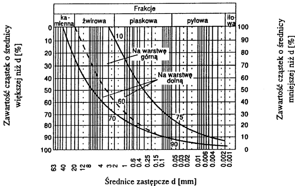
Rys. 1. Obszar uziarnienia optymalnej mieszanki gliniasto-żwirowej
