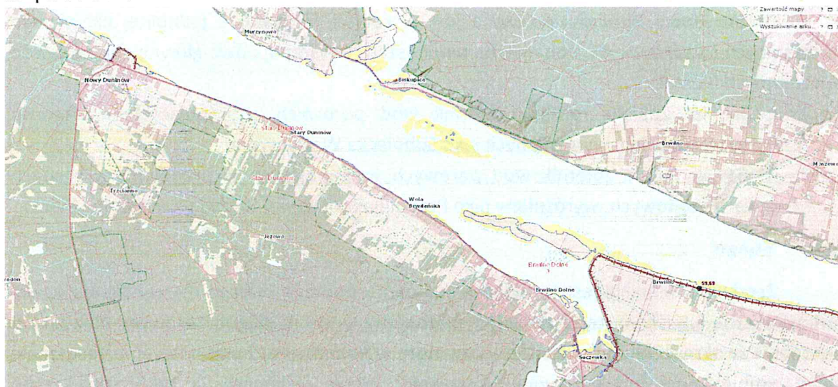
Rysunek 5. Obszary ryzyka powodziowego 1% (kolor żółty) na terenie gminy Nowy Duninów
