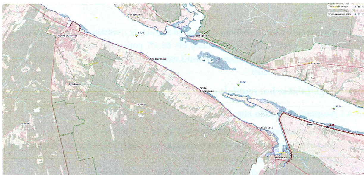
Rysunek 6. Obszary zagrożenia powodziowego (kolor granatowy) z głębokością wody 1m, raz na 100 lat w obrębie miejscowości Nowy Duninów i Soczewka
