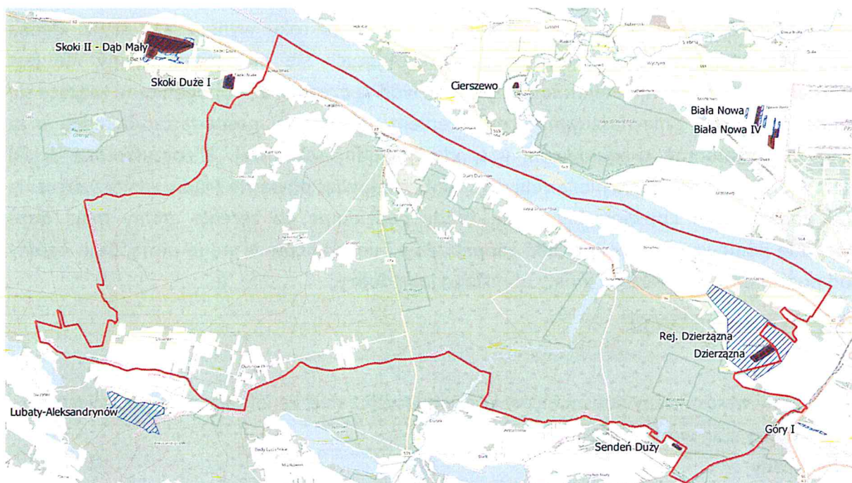
Rysunek 8. Złoża kopalin (kolor niebieski) oraz tereny górnicze (brązowy) na tle gminy Nowy Duninów Źródło: opracowanie własne na podstawie danych Państwowego Instytutu Geologicznego
